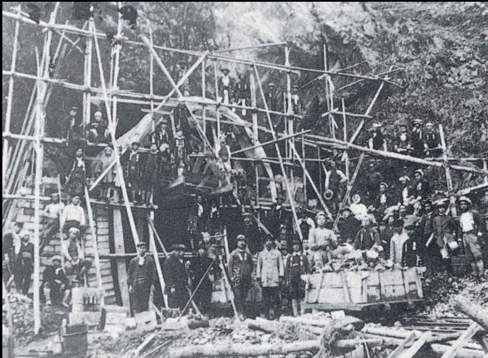
工事中の高山線のトンネル －大正9年9月 撮影場所不明－ 図説可児・加茂の歴史から
